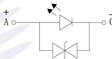
Fig.1-4 Polarity 极性
