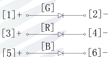
Fig. 1-4 Polarity 极性
