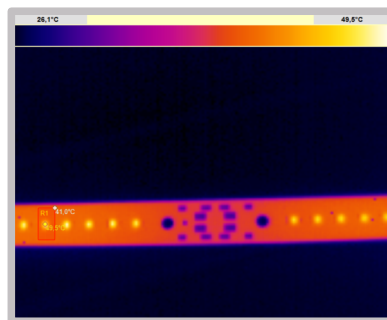
Термограмма, модуль NEO-L-48LS2835_448 ток 350 мА, T_a = 25^\circ\text{C} , установившийся тепловой режим, без радиатора.
