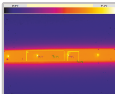
Термограмма, модуль NEO-L-18LS2835 ток 350 mA, T_a = 25^\circ\text{C} , установившийся тепловой режим, без радиатора.
