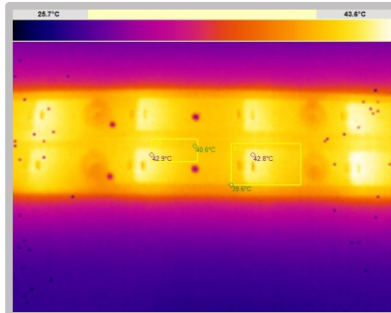
Термограмма, модули NEO-L-18LS2835-490x14 ток 300 мА, Ta = 25°C, установившийся тепловой режим, без радиатора.
