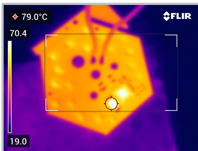
Термограмма NEO-H-18LS2835-AC Питание от сети 230В 60Гц, T_a = 25^\circ\text{C} , установившийся тепловой режим, радиатор STEP-71
