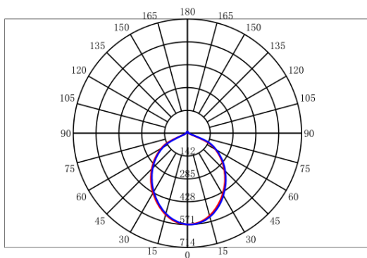
配光曲线
