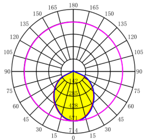
配光曲线
