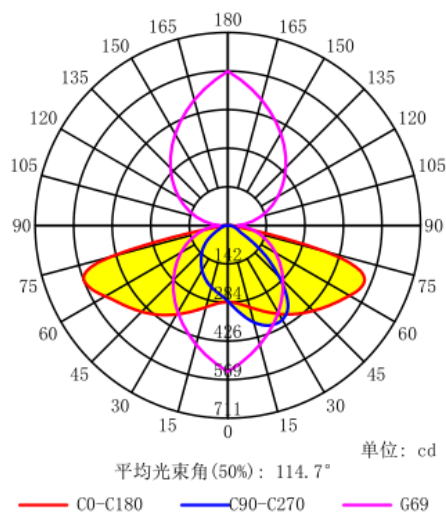
配光曲线
