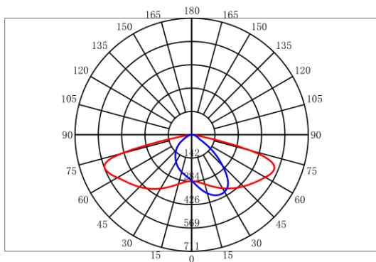
配光曲线
