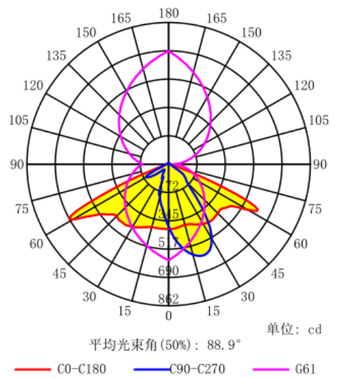
配光曲线
