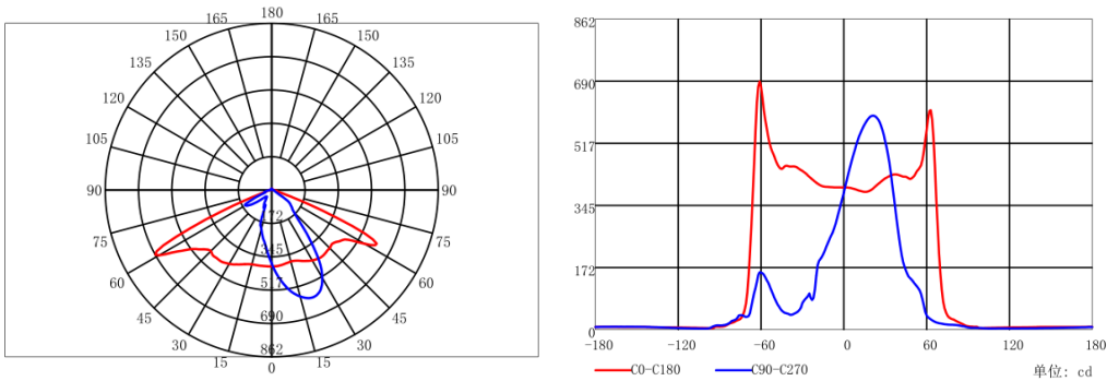
配光曲线
