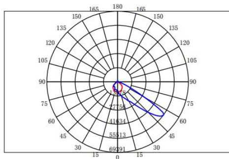
配光曲线
