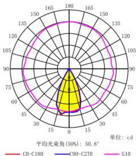
配光曲线
