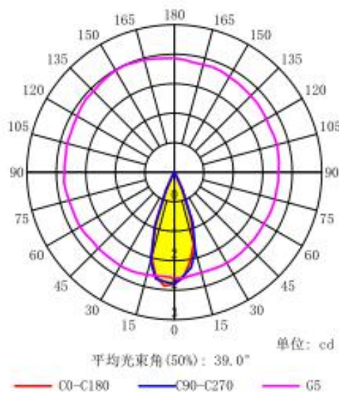
配光曲线
