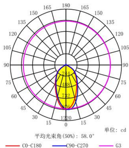
配光曲线
