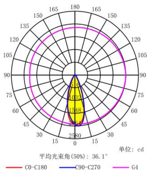
配光曲线
