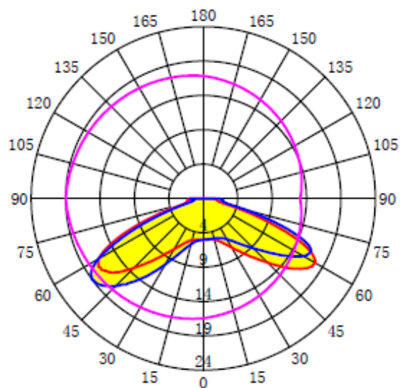
配光曲线
