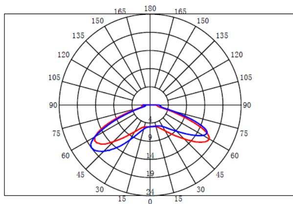
配光曲线
