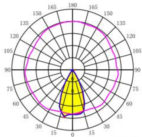
配光曲线
