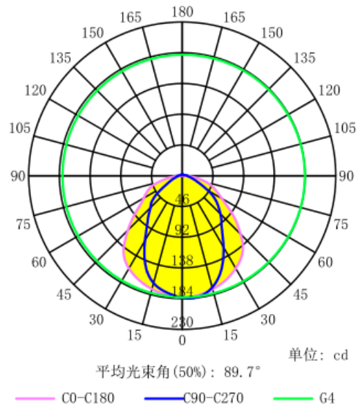
配光曲线
