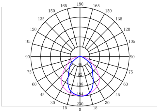
配光曲线
