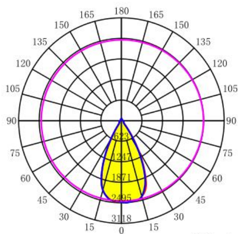
配光曲线
