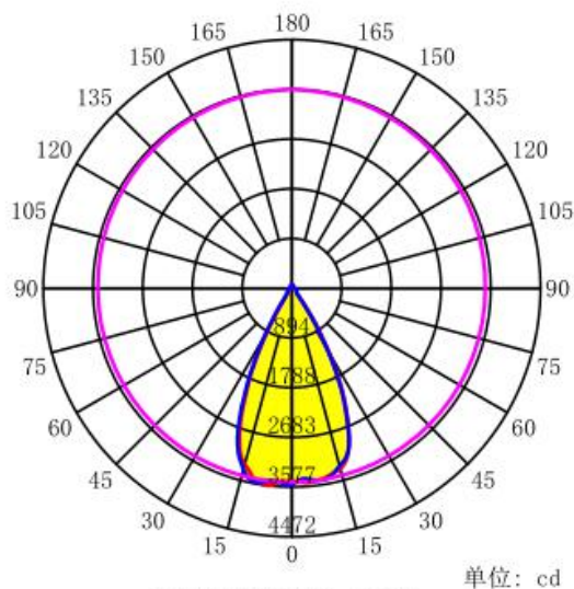
配光曲线
