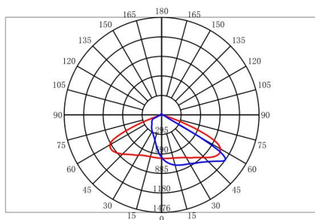
配光曲线
