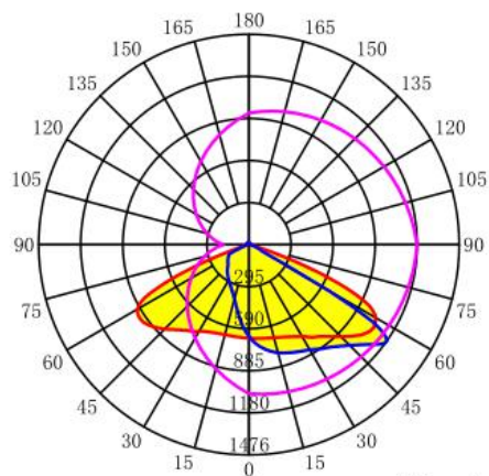
配光曲线
