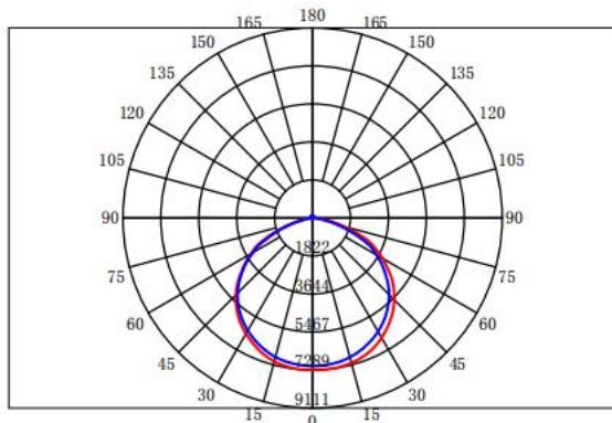
配光曲线
