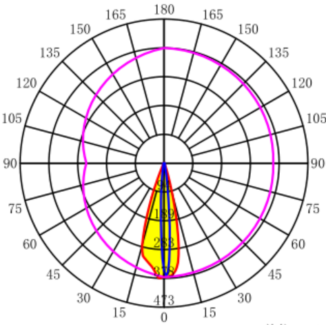
配光曲线
