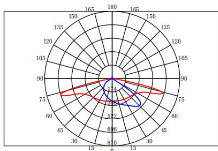
配光曲线
