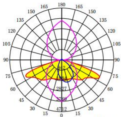
配光曲线
