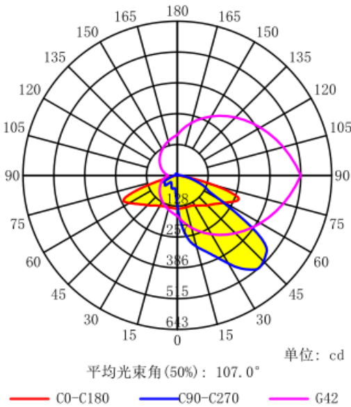
配光曲线
