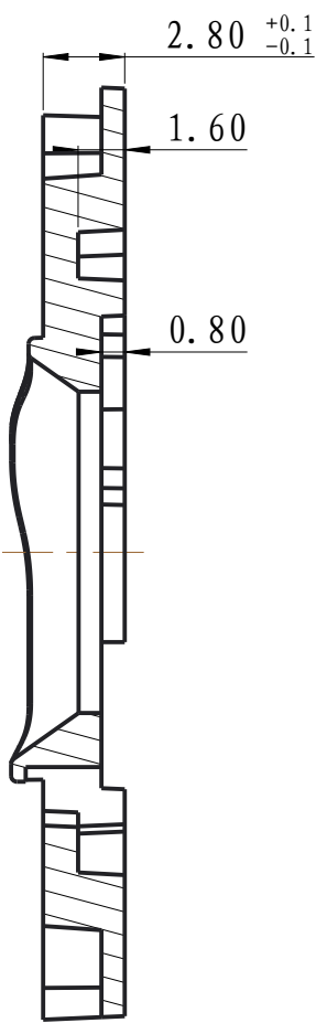
截面 XSEC0001-XSEC0001
